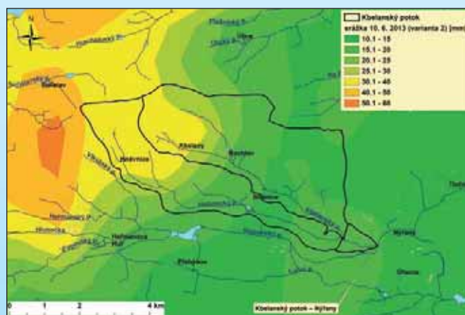
Obr. 2.4 Plošné rozložení srážek (varianta 1 vlevo, varianta 2 vpravo) s vyznačením zasaženého povodí pro 8. 6., 9. 6. a 10. 6. 2013.
