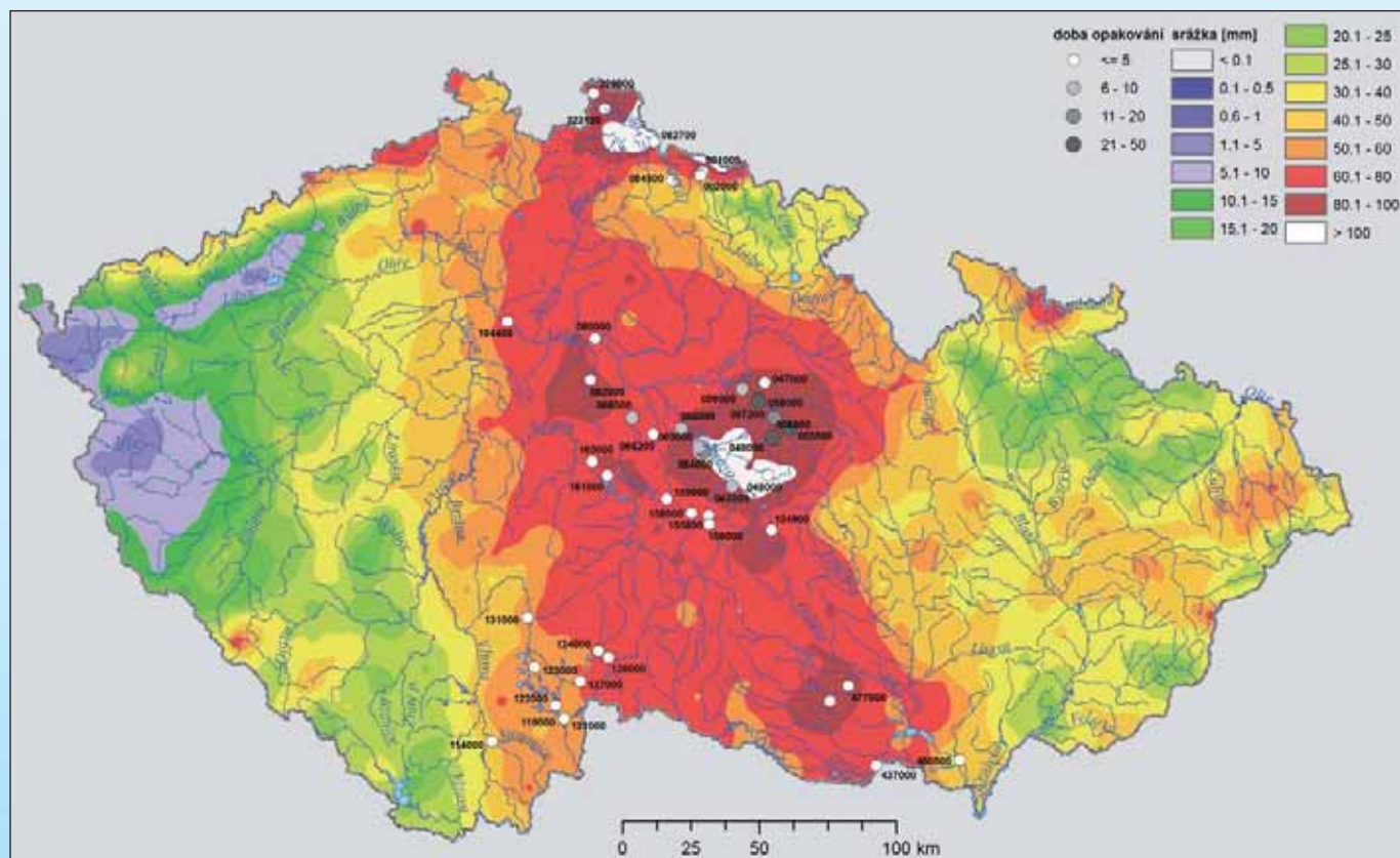
Obr. 1.25 Plošné rozložení srážek vypadlých od 24. června 8:00 do 26. června 8:00 SELČ, společně s vyznačením dob opakování kulminačních průtoků ve vodoměrných stanicích.
